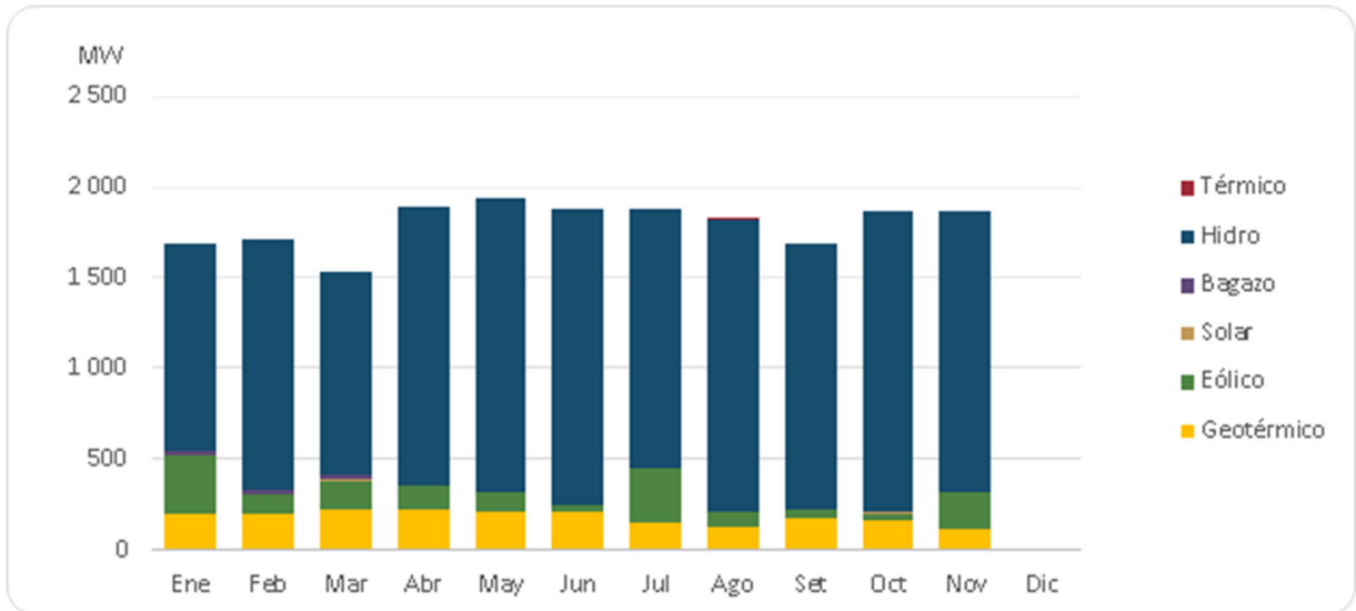
Gráfico 10. Composición de la demanda por fuente a la hora de la máxima enero – noviembre, 2021.
