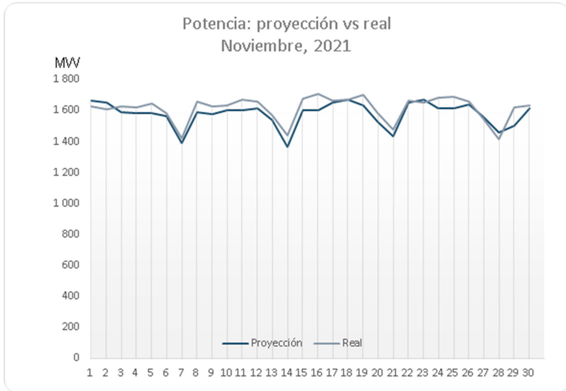
Gráfico 8. Comparación de la demanda de potencia – noviembre, 2021.
