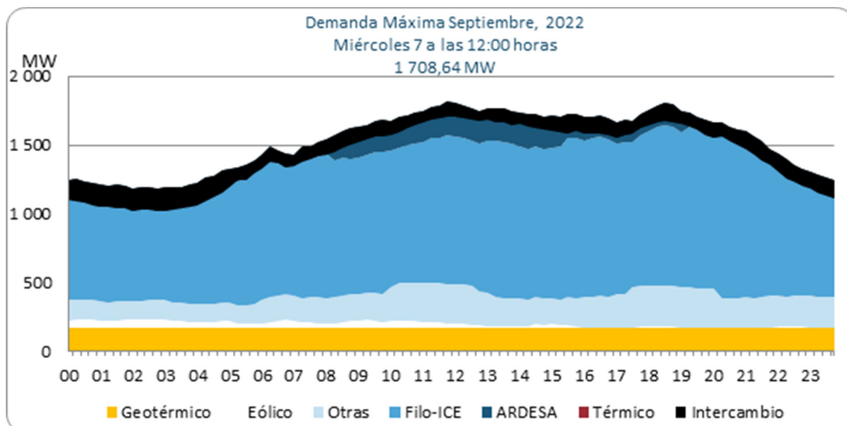
Gráfico 9. Composición de la demanda máxima – septiembre del año 2022, registrada el miércoles 7.
