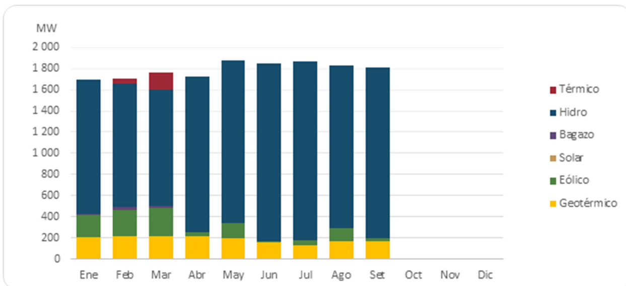
Gráfico 10. Composición de la demanda por fuente a la hora de la máxima enero – septiembre, 2022.
