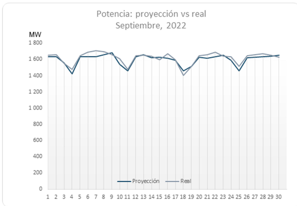
Gráfico 8. Comparación de la demanda de potencia – septiembre, 2022.
