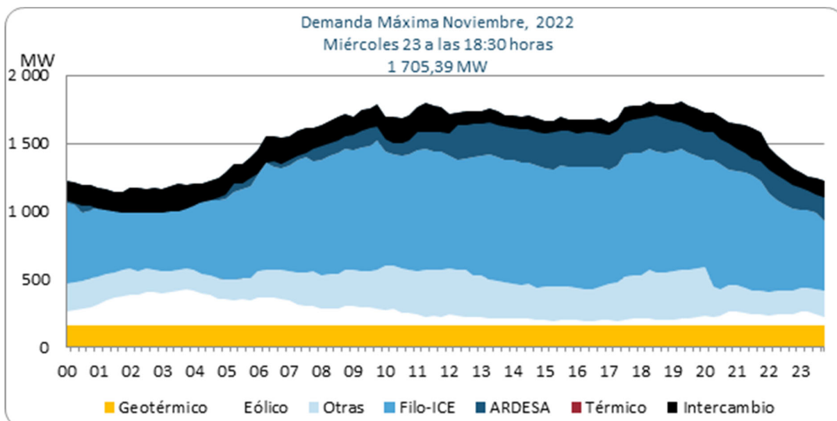
Gráfico 9. Composición de la demanda máxima – noviembre del año 2022, registrada el miércoles 23.
