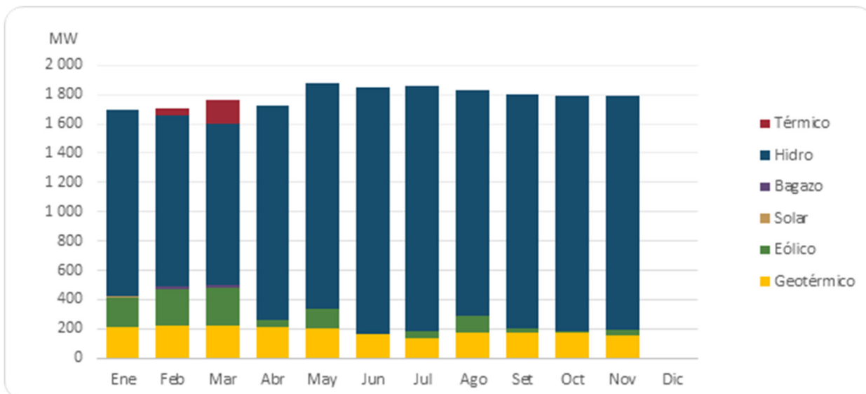
Gráfico 10. Composición de la demanda por fuente a la hora de la máxima enero – noviembre, 2022.
