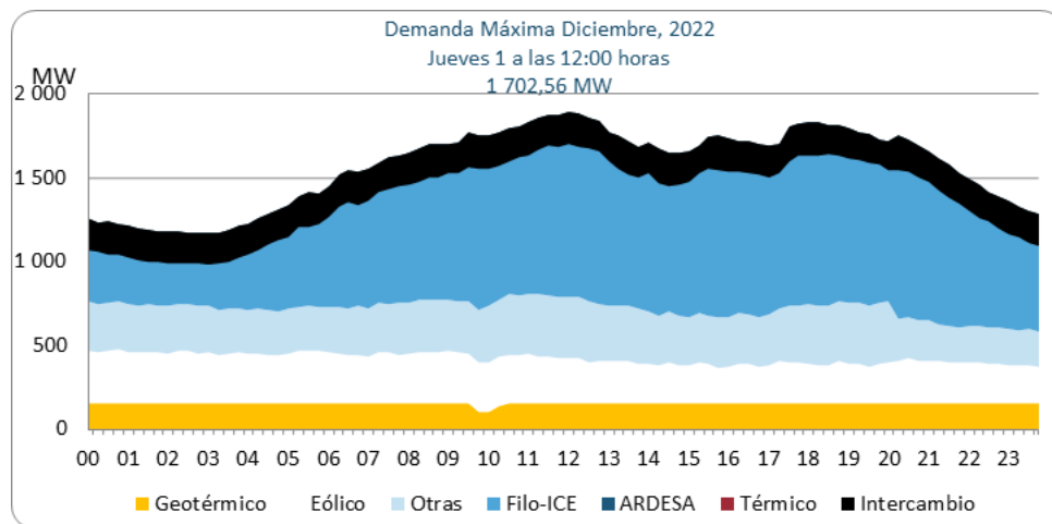
Gráfico 9. Composición de la demanda máxima – diciembre del año 2022, registrada el jueves 1.
