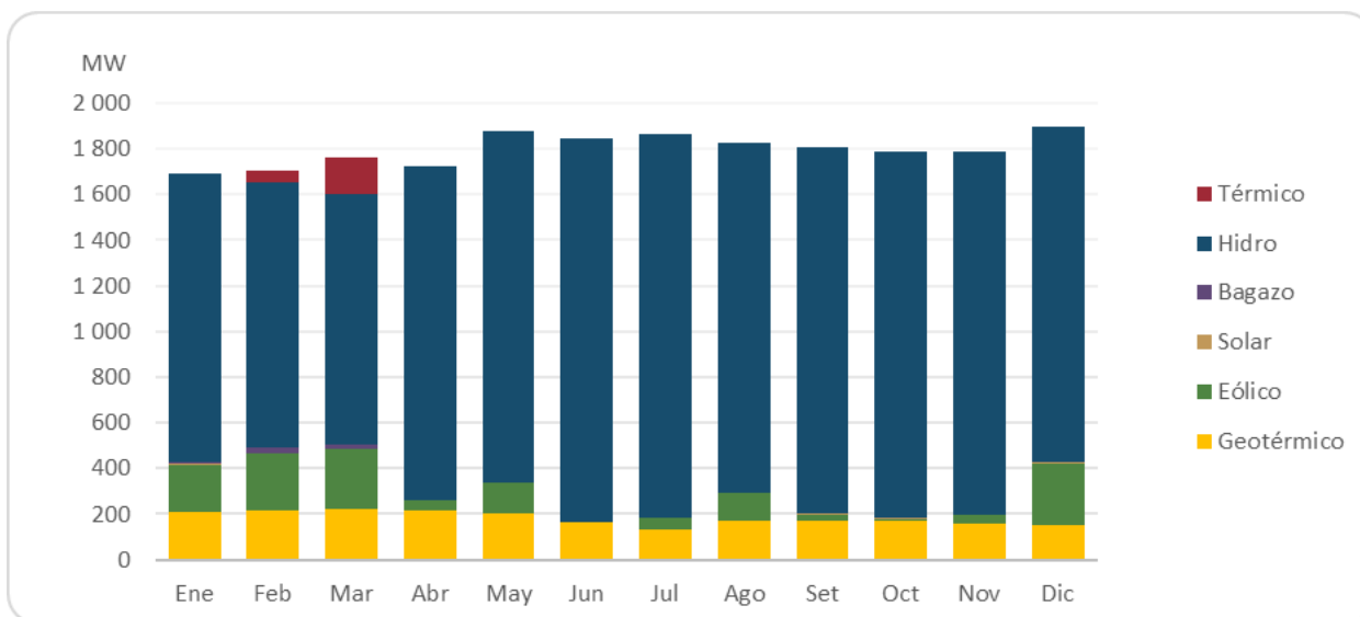
Gráfico 10. Composición de la demanda por fuente a la hora de la máxima enero – diciembre, 2022.
