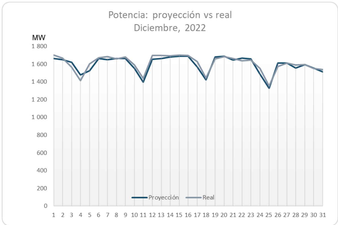
Gráfico 8.Comparación de la demanda de potencia – diciembre, 2022.
