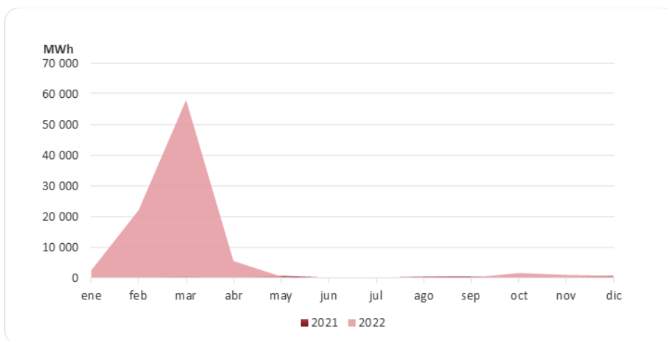
Gráfico 6. Comparación de generación termoeléctrica 2021 - 2022.
