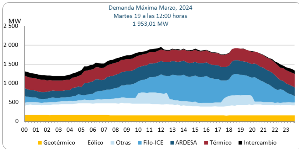
Gráfico 9. Composición de la demanda máxima – marzo del año 2024, registrada el martes 19.
