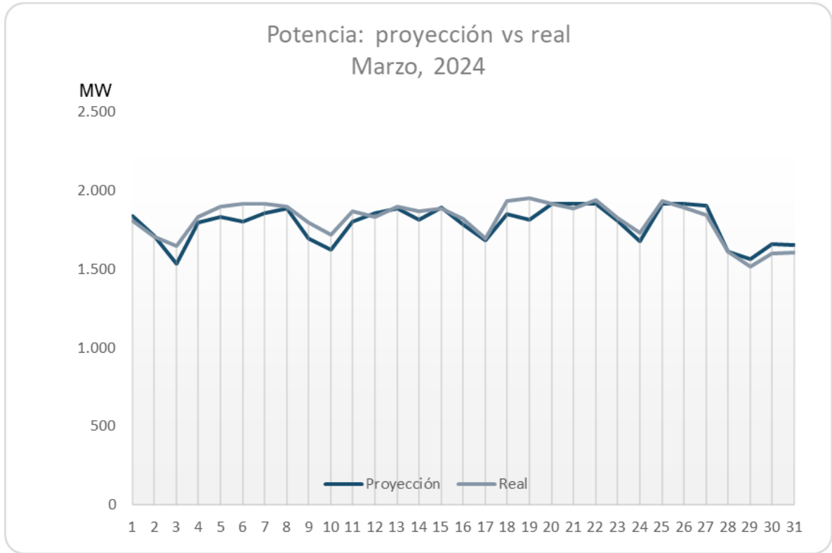
Gráfico 8. Comparación de la demanda de potencia – marzo, 2024.
