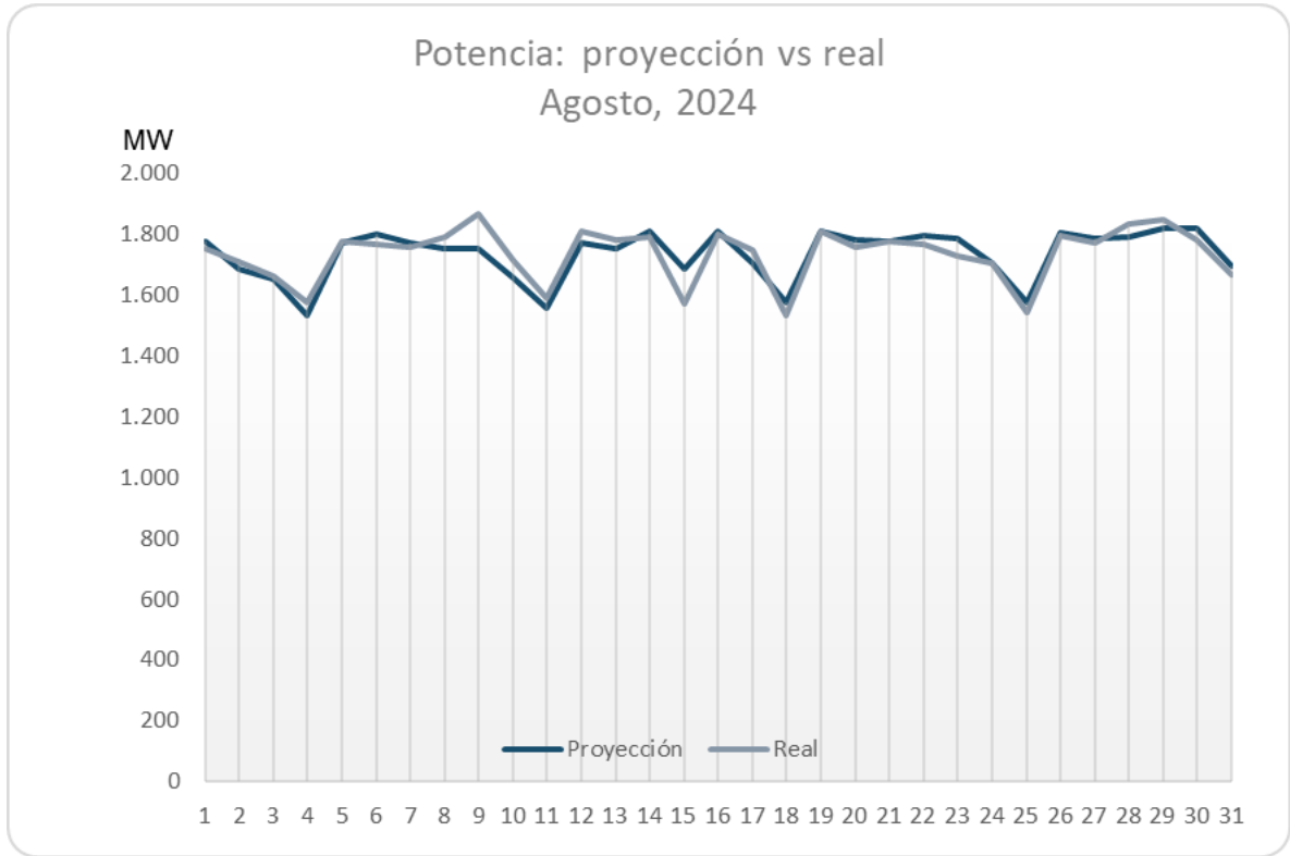
Gráfico 8. Comparación de la demanda de potencia – agosto, 2024.
