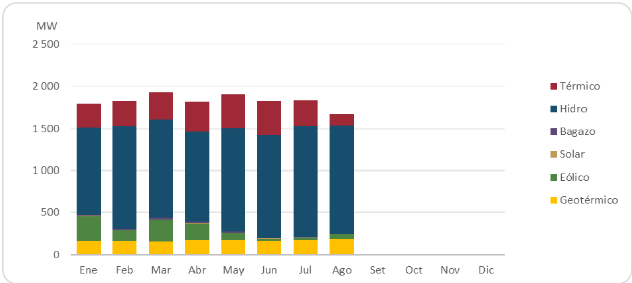
Gráfico 10. Composición de la demanda por fuente a la hora de la máxima enero – agosto, 2024.
