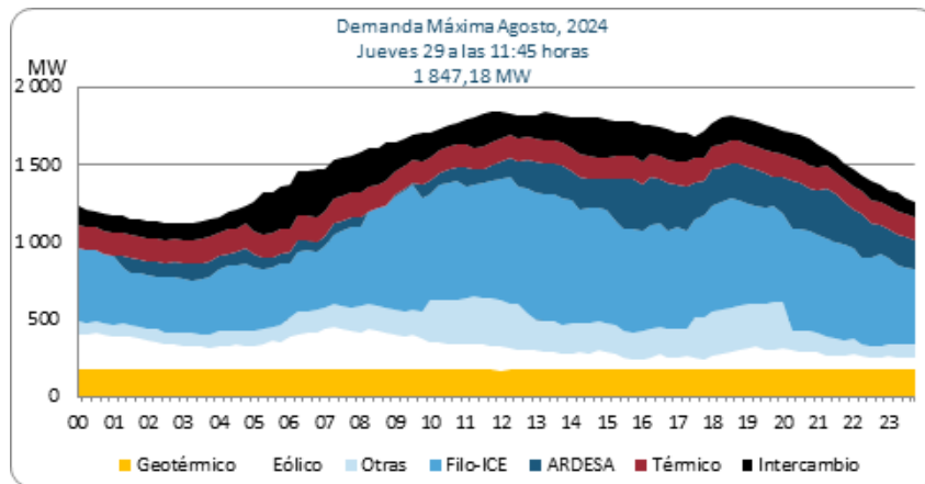
Gráfico 9. Composición de la demanda máxima – agosto del año 2024, registrada el viernes 9.
