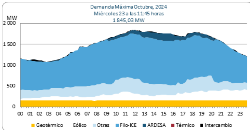
Gráfico 9. Composición de la demanda máxima – octubre del año 2024, registrada el miércoles 23.
