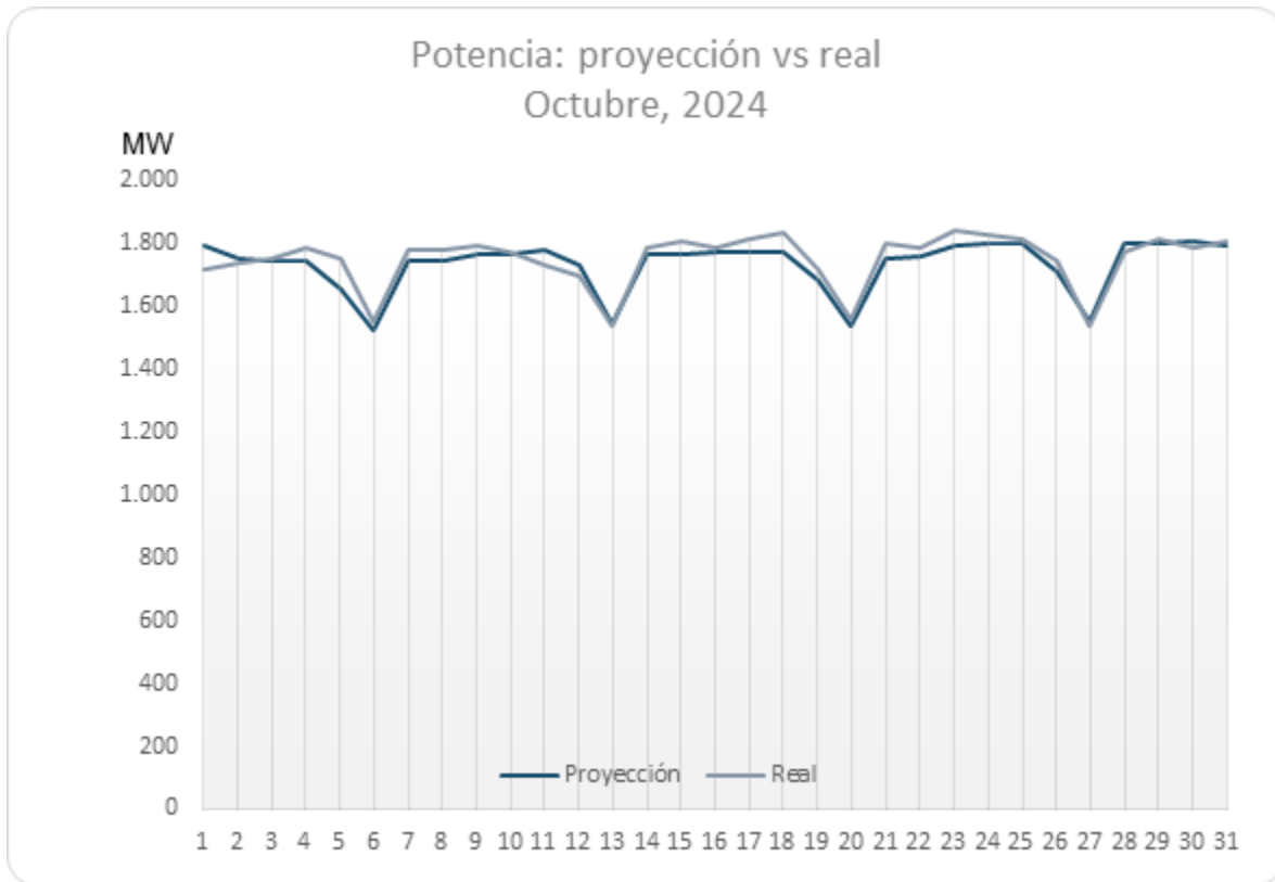
Gráfico 8. Comparación de la demanda de potencia – octubre, 2024.
