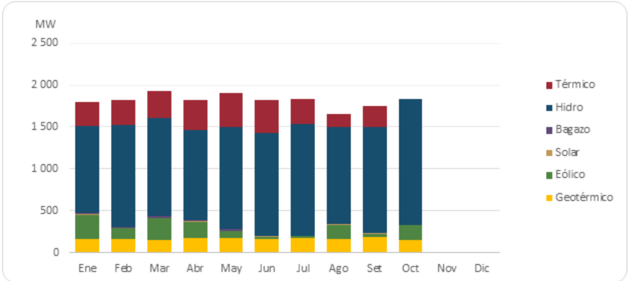
Gráfico 10. Composición de la demanda por fuente a la hora de la máxima enero – octubre, 2024.
