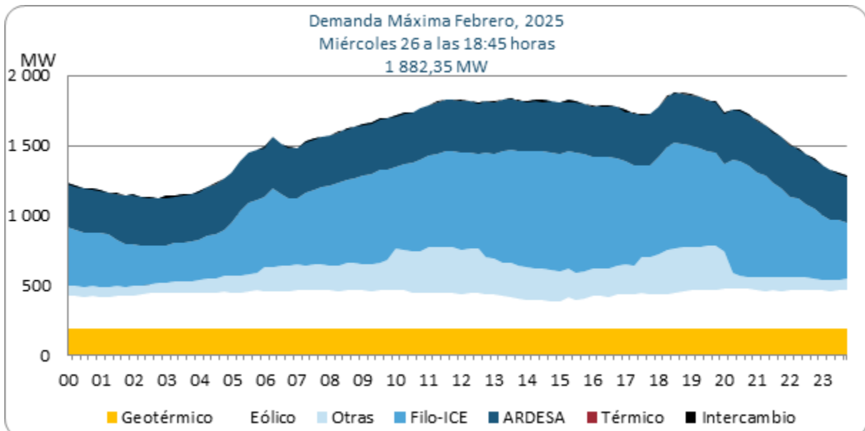
Gráfico 9. Composición de la demanda máxima – febrero del año 2025, registrada el miércoles 26.
