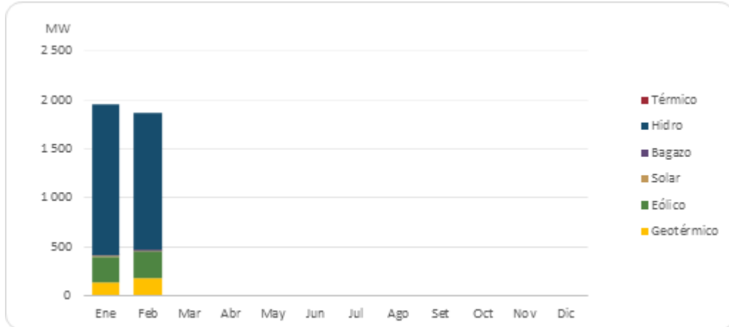
Gráfico 10. Composición de la demanda por fuente a la hora de la máxima enero – febrero, 2025.
