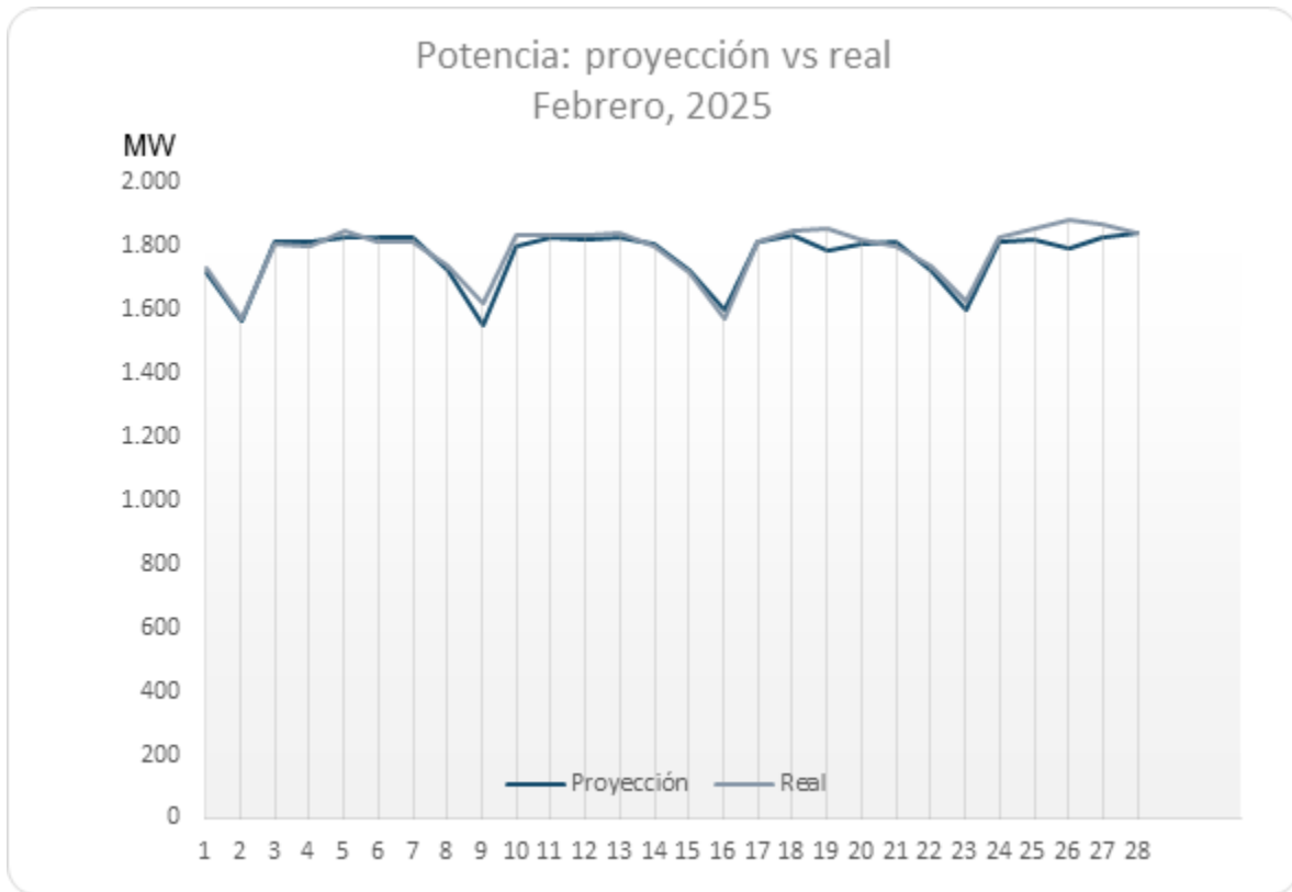
Gráfico 8. Comparación de la demanda de potencia – febrero, 2025.
