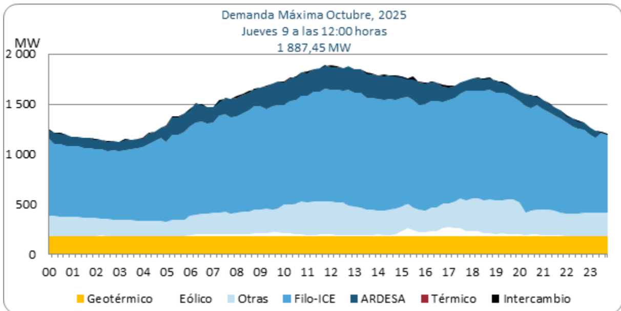
Gráfico 9. Composición de la demanda máxima – octubre del año 2025, registrada el jueves 9.
