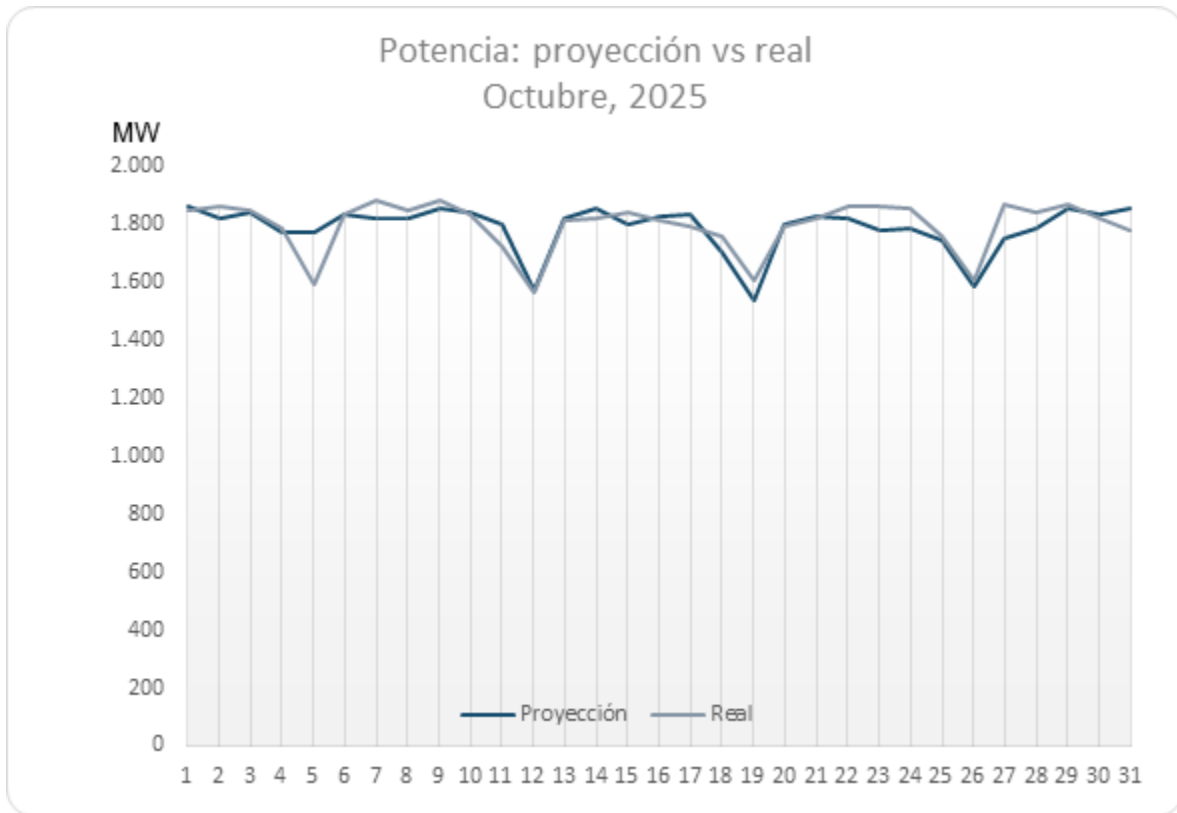
Gráfico 8. Comparación de la demanda de potencia – octubre, 2025.
