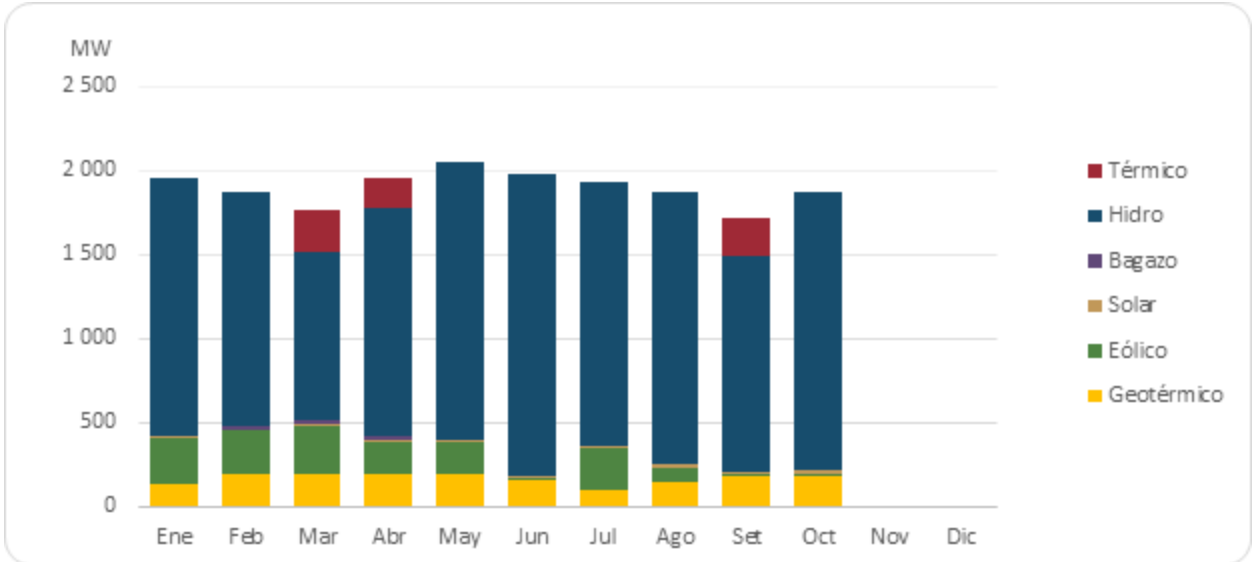
Gráfico 10. Composición de la demanda por fuente a la hora de la máxima enero – octubre, 2025.
