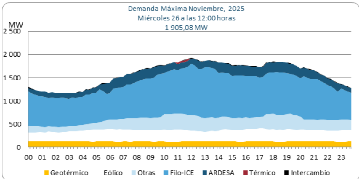
Gráfico 9. Composición de la demanda máxima – noviembre del año 2025, registrada el miércoles 26.
