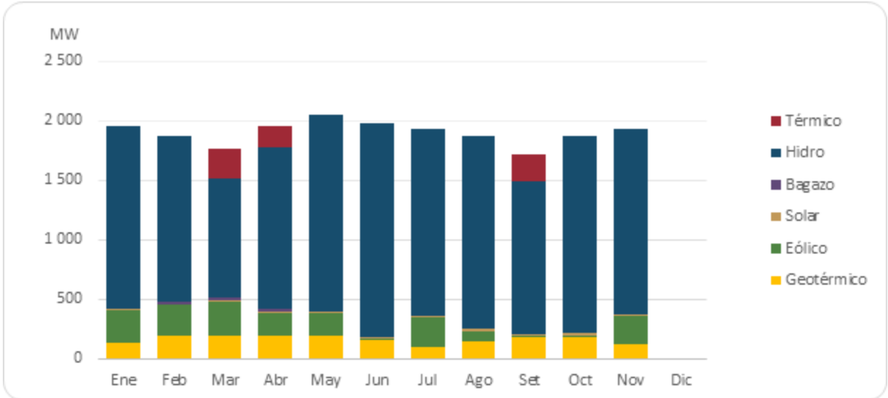
Gráfico 10. Composición de la demanda por fuente a la hora de la máxima enero – noviembre, 2025.
