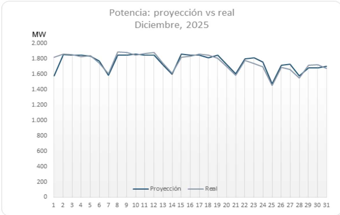
Gráfico 8. Comparación de la demanda de potencia – diciembre, 2025.
