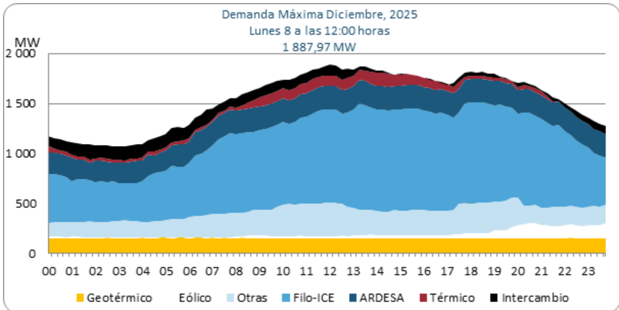
Gráfico 9. Composición de la demanda máxima – diciembre del año 2025, registrada el lunes 8.
