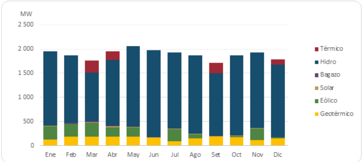
Gráfico 10. Composición de la demanda por fuente a la hora de la máxima enero – diciembre, 2025.
