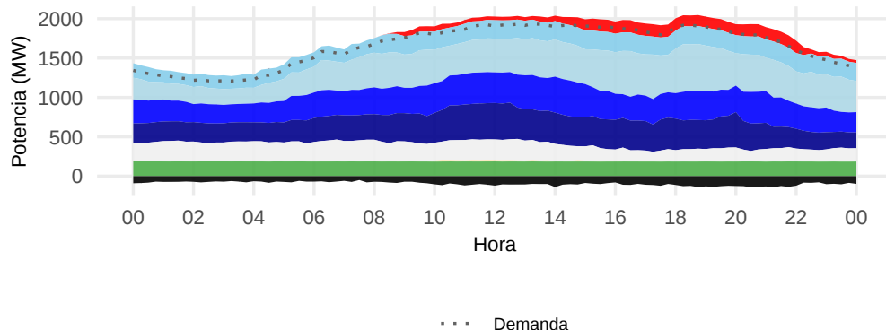
Figura 1: Demanda nacional, generación por fuente e intercambios
