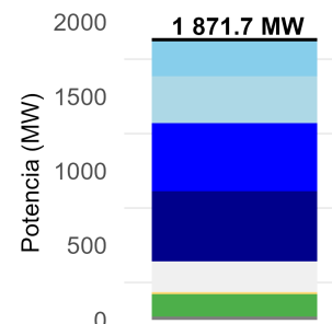
Figura 2: Composición de la generación a la hora de la máxima demanda considerando intercambios
